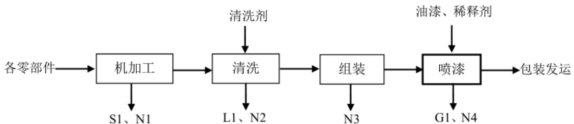
图 4-1 减速设备及变频器加工生产流程图
