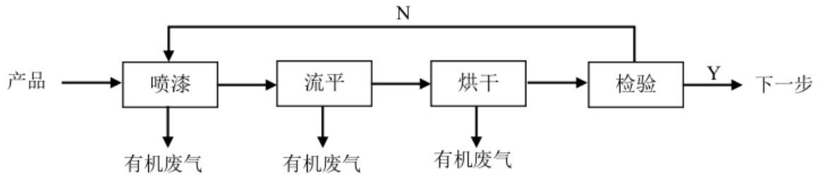
图 4-2 喷漆工艺流程图
