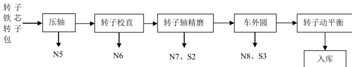
图 4-3 转子加工流程图
